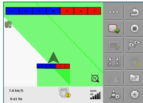
Ohne ISOBUS-Jobrechner: SECTION-View in der Kopfzeile und als Arbeitsbalken
