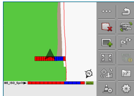
Mit einem ISOBUS-Jobrechner: SECTION-View in der Fußzeile und als Arbeitsbalken
