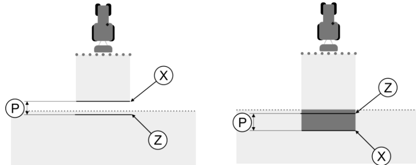
Linien für den Parameter "Trägheit Korrektur bei Ein". Links: Feldspritze schaltet zu spät ein. Rechts: Feldspritze schaltet zu früh ein.
