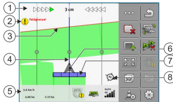
Arbeitsmaske während der Arbeit
