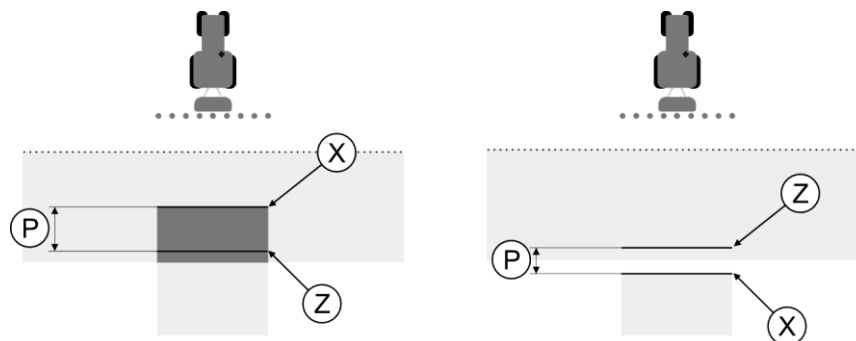
Linien für den Parameter "Trägheit Korrektur bei Aus". Links: Feldspritze schaltet zu spät aus. Rechts: Feldspritze schaltet zu früh aus.
