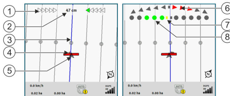
Bildschirm-Lightbar. links: Textmodus; rechts: Grafikmodus
