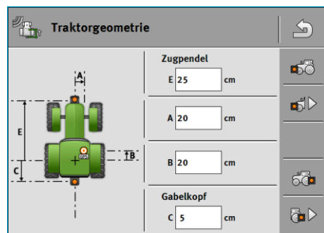
Beispielhafte Traktorgeometrie
