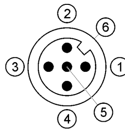
Pinbelegung des Steckers
