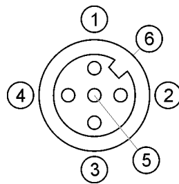
Pinbelegung der Buchse (im Terminal)
